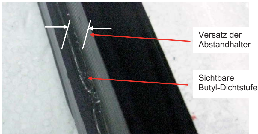
Abbildung 4 Verformung des Randverbunds
