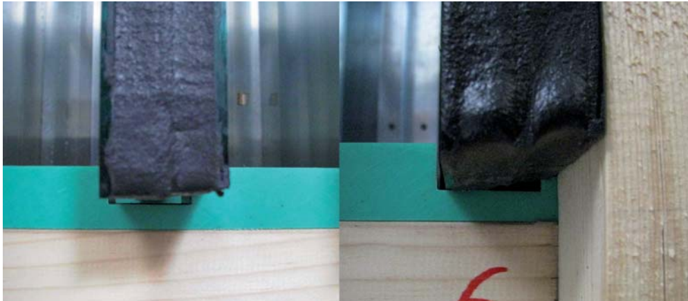
Abbildung 3 Links: PU-Randverbund, rechts: Polysulfid-Randverbund
